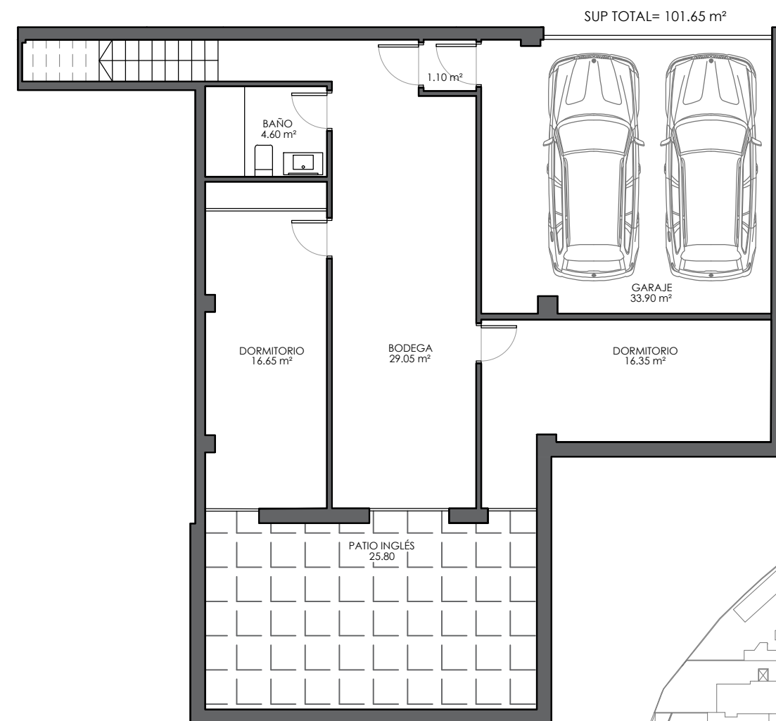
PLANTA SÓTANO
