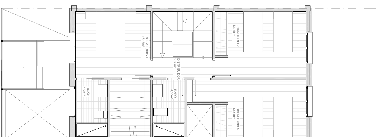
PLANTA PRIMERA
