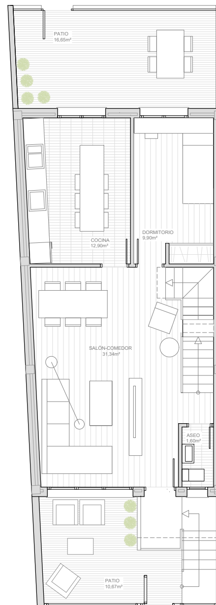
PLANTA BAJA
