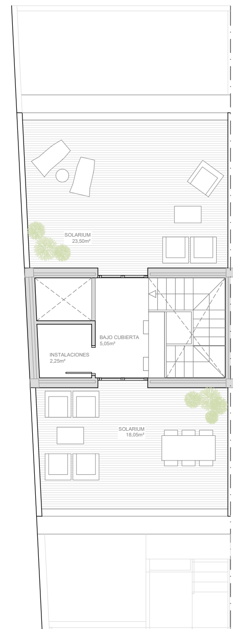
PLANTA SOLARIUM
