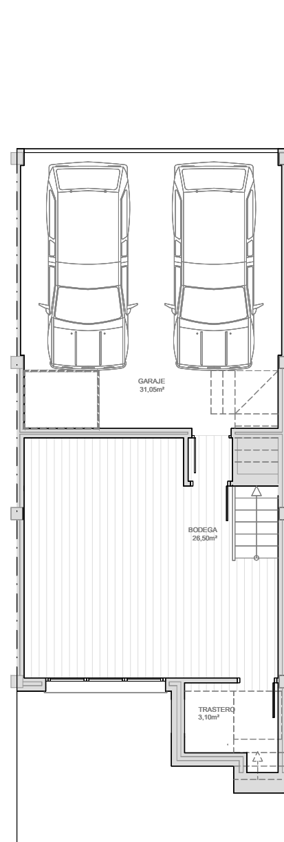
PLANTA SEMISÓTANO
