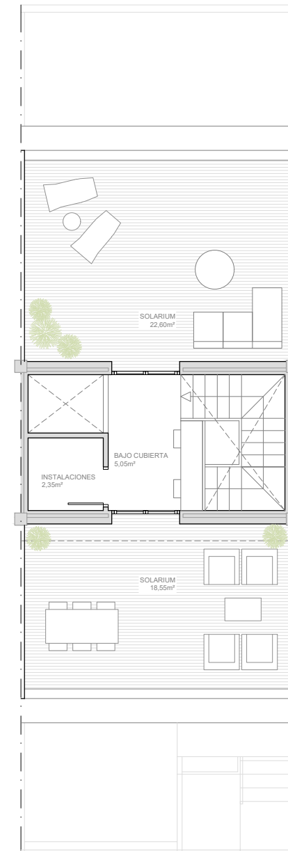
PLANTA SOLARIUM
