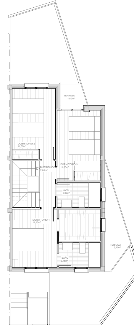
PLANTA PRIMERA
