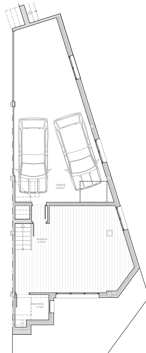
PLANTA SEMISÓTANO
