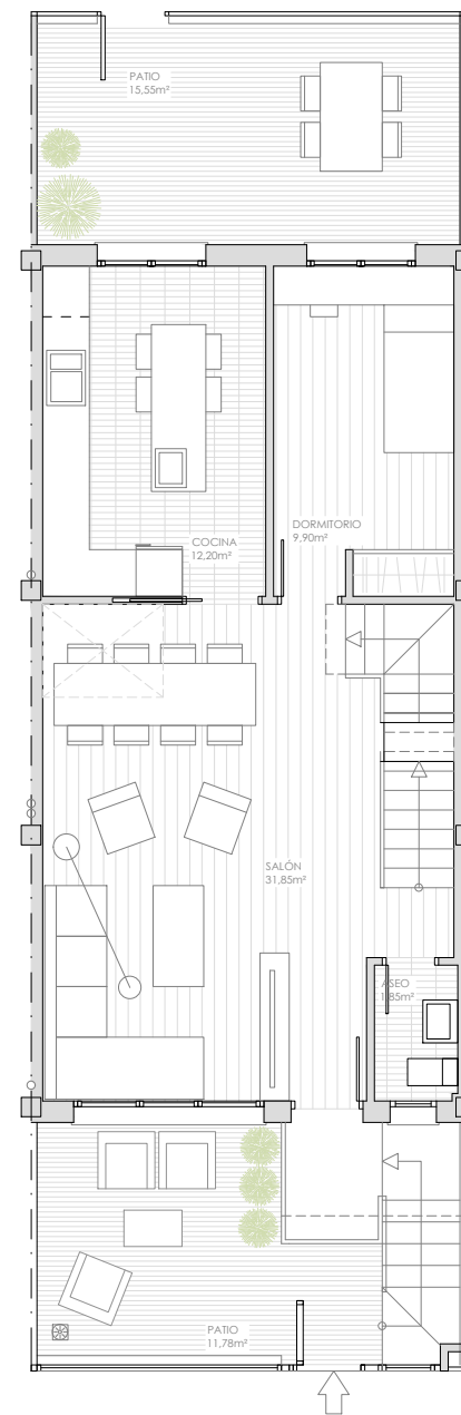
Planta baja
