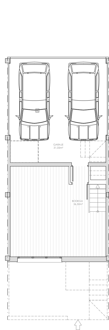
Planta semisótano
