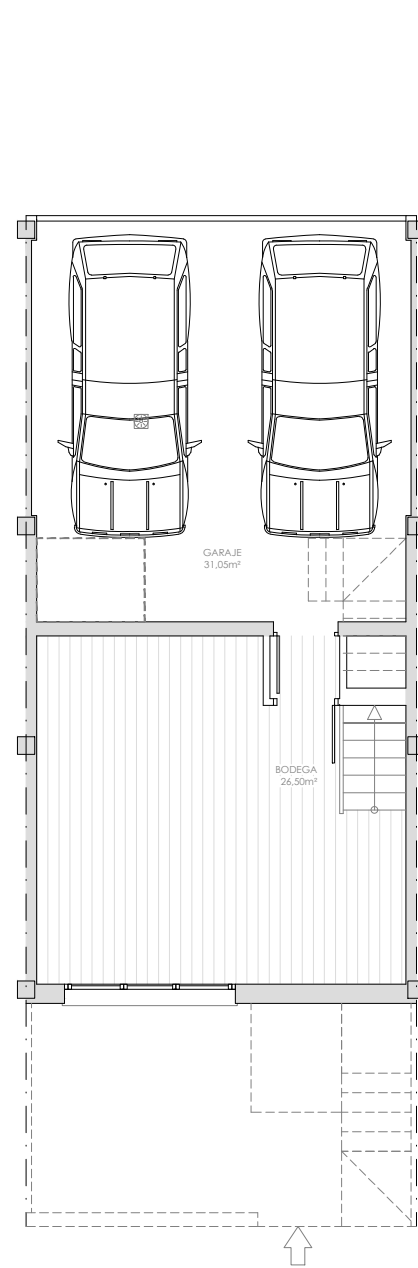
Planta semisótano
