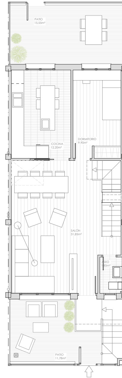
Planta baja
