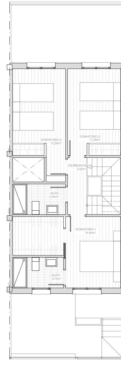
Planta primera
