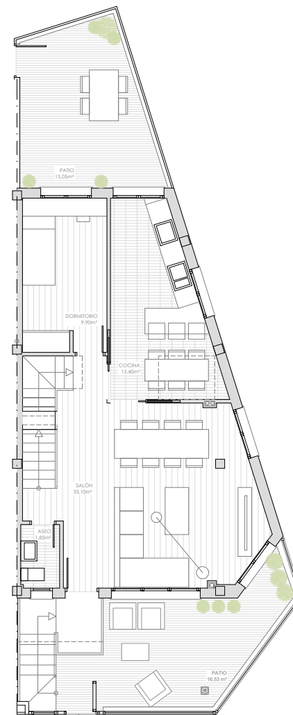
Planta baja
