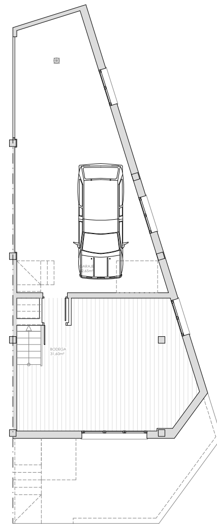
Planta semisótano
