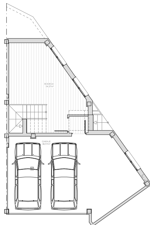
Planta semisótano
