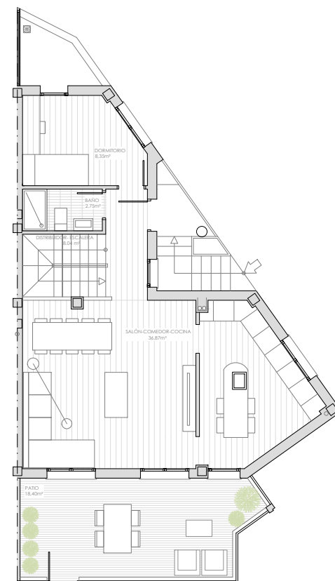
Planta baja
