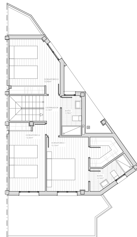
Planta primera
