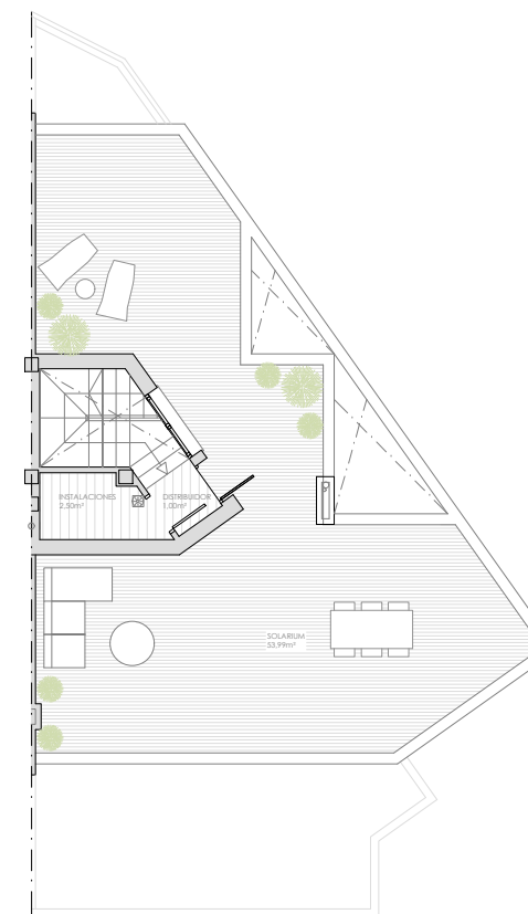
Planta casetón
