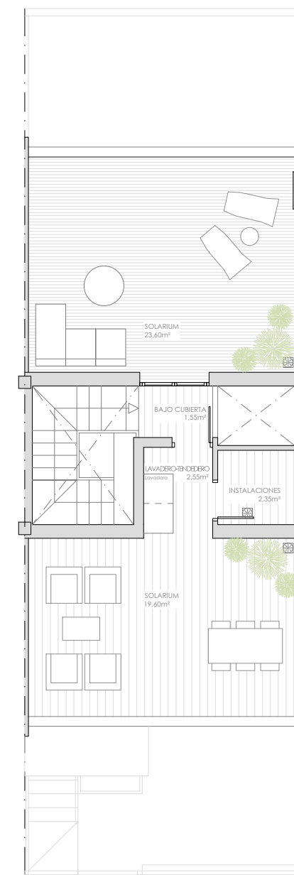
Planta casetón
