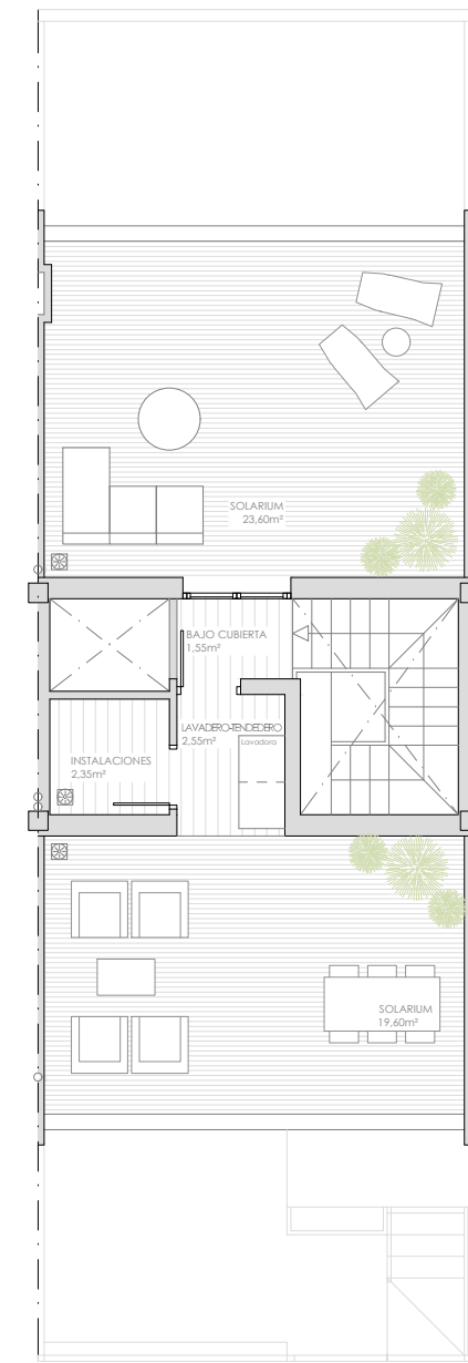
Planta casetón
