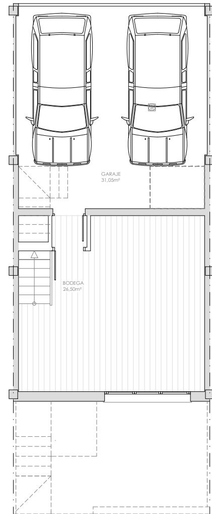
Planta semisótano
