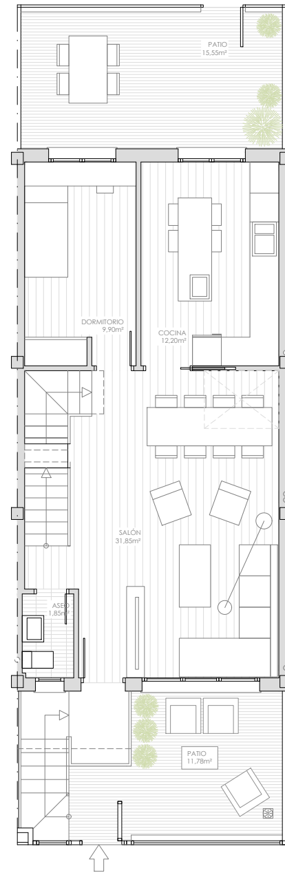
Planta baja
