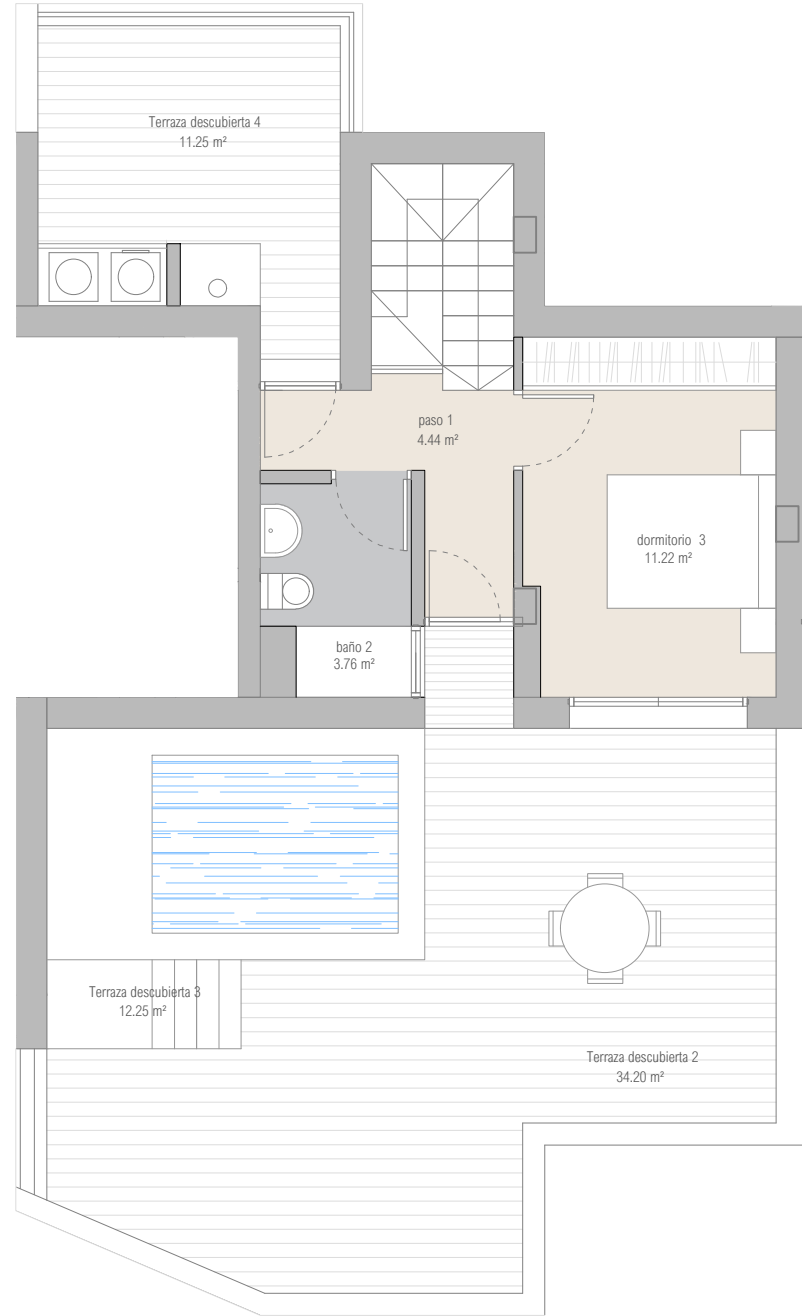
Planta cubierta
